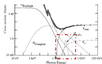
Sezione d'urto per reazioni fotonucleari: Esempio di risonanza gigante in Piombo, picco a 13,6 MeV
